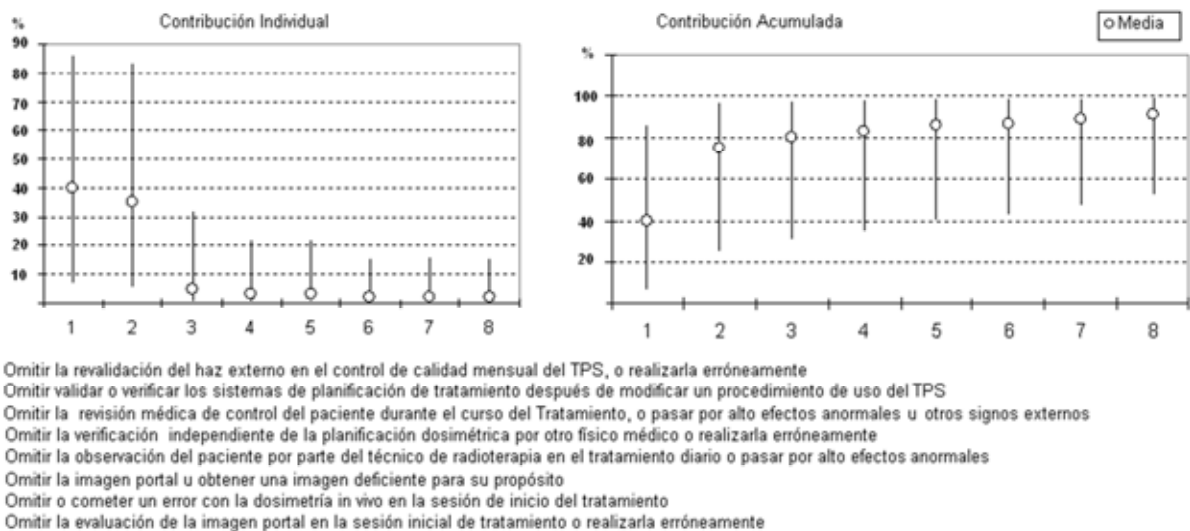
FIG. 6. Incertidumbres de los valores de importancia Fussell Vesely aplicada a las barreras que provocan exposiciones accidentales de múltiples pacientes.
